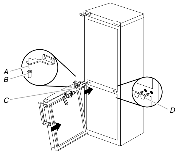
A. Center hinge pin B. Bushing
